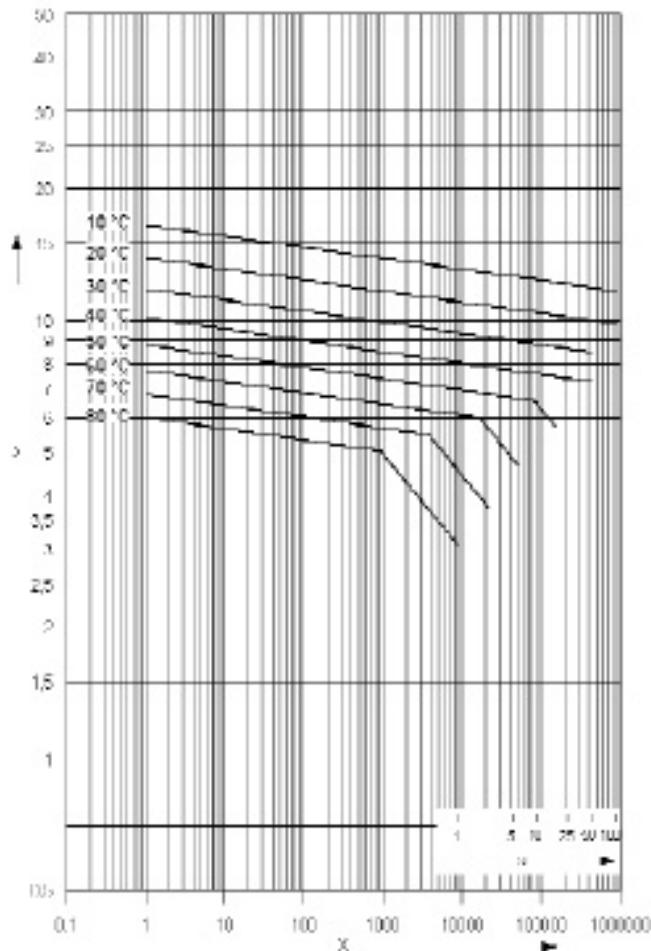
Рис. 2. Пример нормированной температурно-временной зависимости прочности полимерного материала
